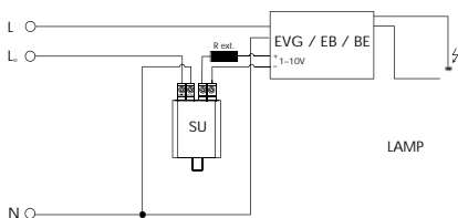
Schaltbild SU 1-10 V K
